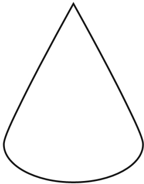
Cone
